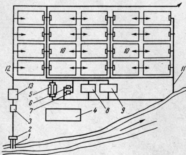
Рис. 8. Схема осетрового рыбодоводного завода: 1 — водозабор; 2 — насосная станция; 3 — отстойник; 4 — хозяйственный центр; 5 — садки Б. Н. Казанского; 6 — инкубационный цех; 7 — олигохетник; 8 — дафниевые бассейны; 9 — бассейны ВНИРО; 10 — пруды; 11 — сбросная сеть; 12 — водоподающая сеть; 13 — напорный бассейн.
