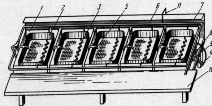
Рис. 17. Инкубационный аппарат конструкции П. С. Ющенко: 1 — наружный ящик; 2 — внутренний ящик; 3 — лопасть; 4 — тяга; 5 — водоподающий кран; 6 — подвижная рама; 7 — борт; 8 — водоподающая труба; 9 — водоотводящий лоток; 10 — стол; 11 — регулятор движения лопасти.
