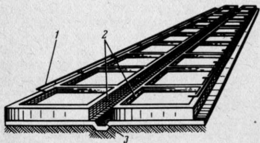
Рис. 33. Дафниевые бассейны: 1 — водоподдающая сеть; 2 — сливное отверстие; 3 — сбросной канал.
