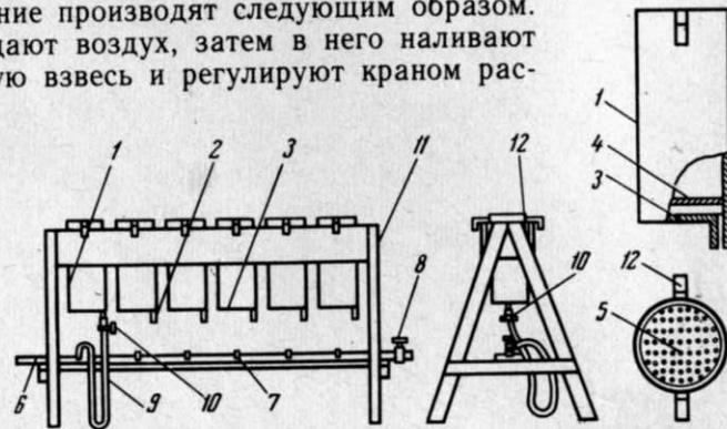
Рис. 16. Схема аппарата Э. В. Орлова для обесклеивания икры и его монтаж в стойке:
