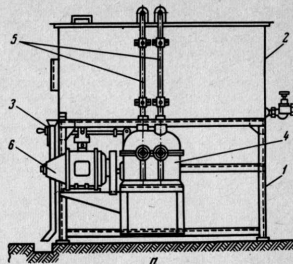
Рис. 18. Инкубационный аппарат конструкции А. Н. Щеколкина;
