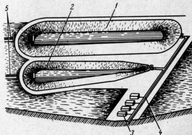
Рис. 9. Садковое хозяйство конструкции Б. Н. Казанского:
