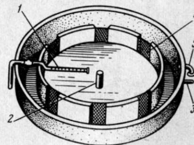
Рис. 23. Бассейн с круговым током воды системы ВНИРО: 1 — «флейта»; 2 — центральный сток; 3 — периферийный сток; 4 — сетка; 5 — аварийный сток.
