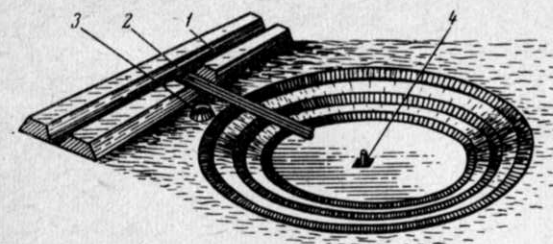
Рис. 26. Грунтовый бассейн с круговым током воды конструкции Аралрыбвода: 1 — водоподводящий канал; 2 — водоподводящий лоток; 3 — бак для дафний; 4 — центральный сток.
